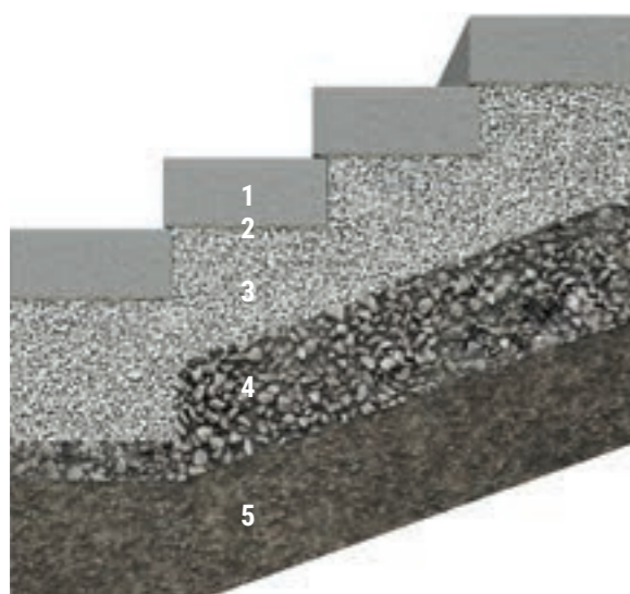
Abbildung 6: Stufenaufbau mit Blocksteinen im Drainbetonbett
