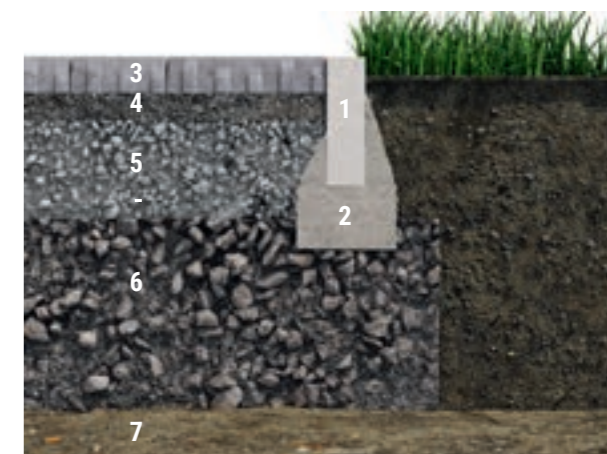
Abbildung 2: Randeinfassung
