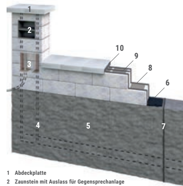
Abbildung 8: Zaunaufbau
